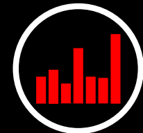
ANALYTIikka & AI
